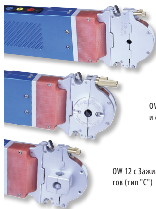
OW 12 с узкой зажимной кассетой (тип "А")
