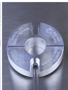
Aluminium-Spanneinsätze zu OW 12, тип "B" (breit) – separat erhältlich
